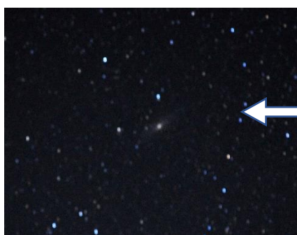
アンドロメダ大星雲
